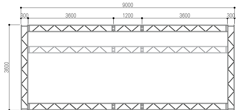
正面
