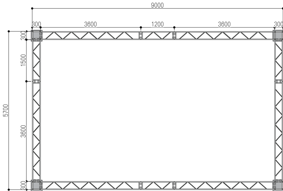
平面
